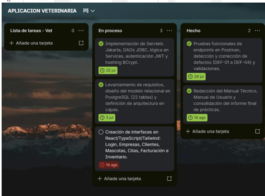
Figura2: Tareas listadas
